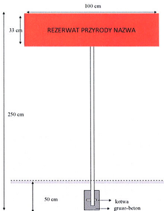
Ryc. Wymiary i sposób montowania tablic informacyjnych z nazwą rezerwatu do gruntu
